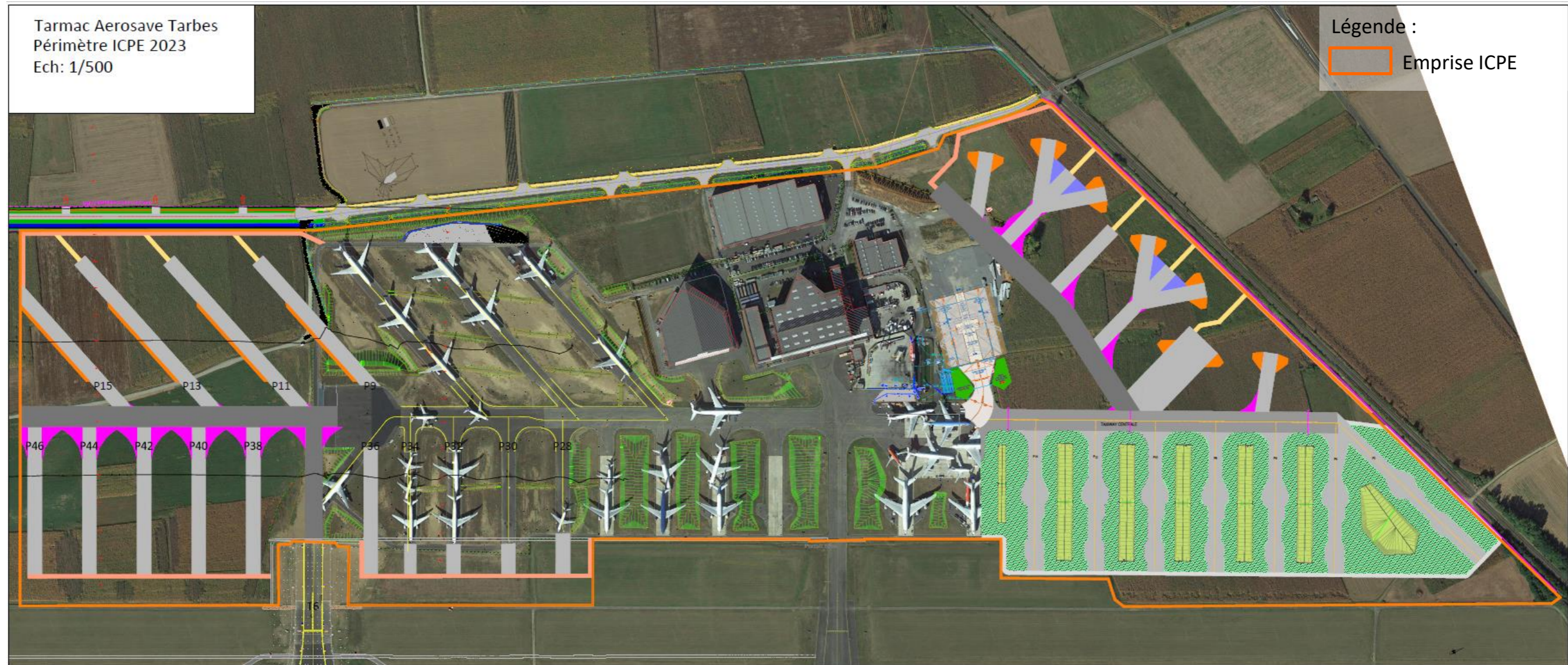
Figure 1 : Plan de masse
